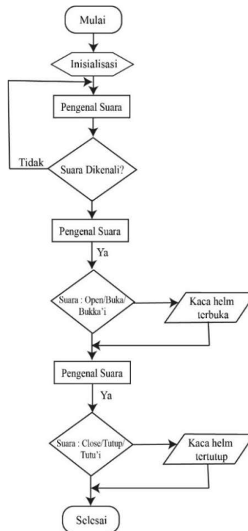
Gambar 4. Flowchart Sistem Buka Tutup Kaca Helm Menggunakan Voice Recognition Module Berbasis Mikrokontroler
