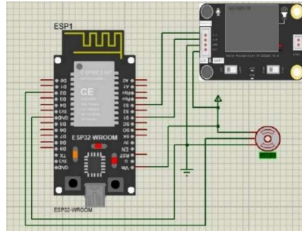
Gambar 2. Rancangan alat Sistem Buka Tutup Kaca Helm Menggunakan Voice Recognition Module Berbasis Mikrokontroler
