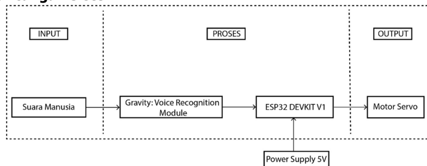
Gambar 1. Diagram Blok Sistem Buka Tutup Kaca Helm Menggunakan Voice Recognition Module Berbasis Mikrokontroler
