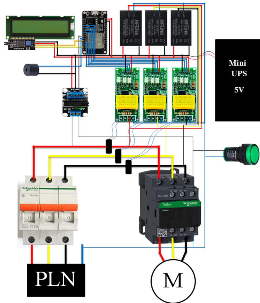
Gambar 2. Rangkaian Sistem Monitoring Tegangan Tiga Phase
